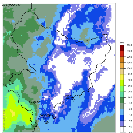
ANTILOPE REANALYSE J+1: lame d'eau sur 01 heure, le 23/09/2024 à 07h00 UTC
