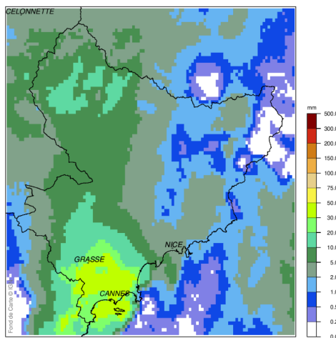
Données horaires de CANNES (06 029 001)
